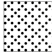
Acoustiroc® ASTRAL 17% Ø2,5 (round, regular) \alpha_w = 0,95 NRC : 0,90
